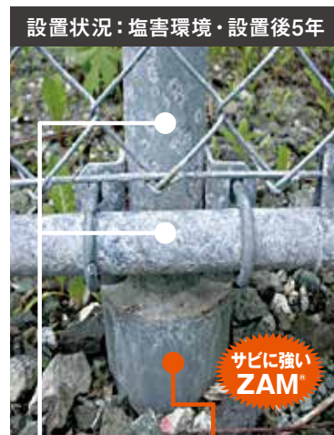
設置状況: 塩害環境・設置後5年 HDZT77(HDZ55) ZAM ® 製鋼管杭
