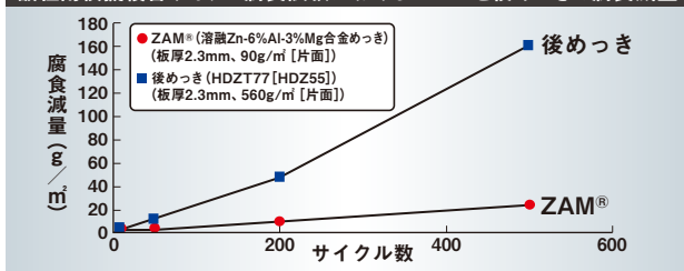
酸性雨模擬複合サイクル腐食試験におけるZAM ® と後めっきの腐食減量
