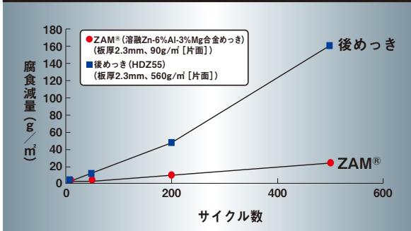
酸性雨模擬複合サイクル腐食試験におけるZAM ® と後めっきの腐食減量
