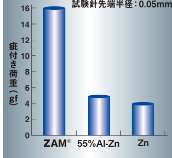
各種めっき鋼板の耐疵付性(スクラッチ試験)
