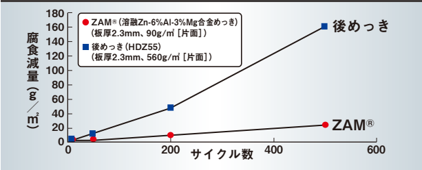
酸性雨模擬曝合サイクル腐食試験におけるZAM ® と後めっきの腐食減量
